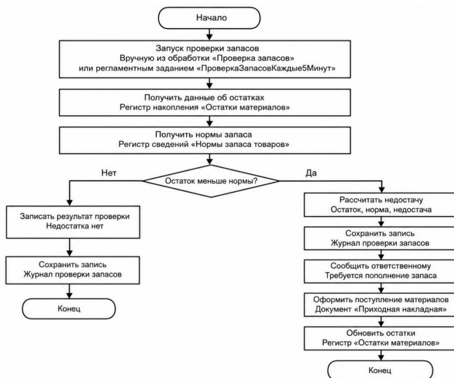
Рисунок 2 – Блок-схема бизнес-процесса контроля остатков
